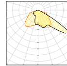
Asimétrico 50° x 110°
