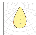
Simétrico 60°
