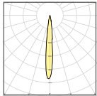
Simétrico 10°
