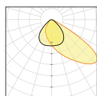
Asimétrico 48° x 92°
