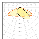
Distribución de la luz ASYM 45° x 140
