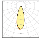
Simétrico 30°
