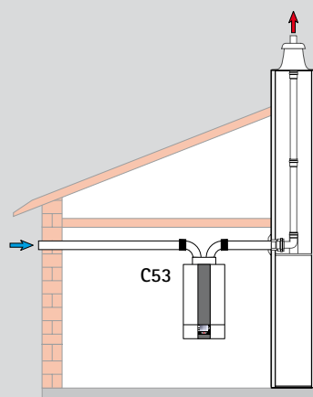
ADAPTADOR DE CONCÉNTRICO A BITUBULAR En polipropileno Alto 250 mm
