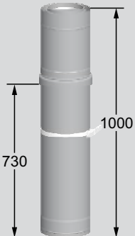
CONDUCTO CONCÉNTRICO PARA PASO DE TEJADO DN250/350 En acero inox./polipropileno Longitud 1000 mm
