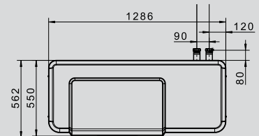
Módulo exterior CHA vista superior
