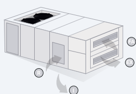
IMPULSIÓN INFERIOR
