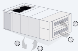
IMPULSIÓN INFERIOR
