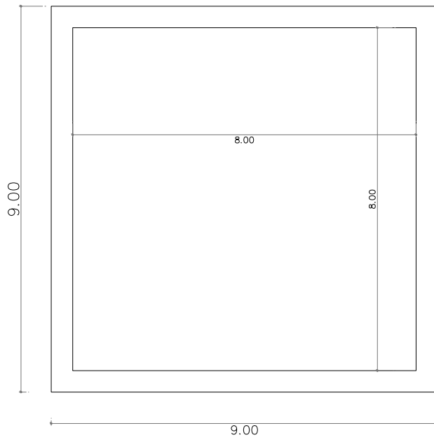
NIVEL CÁMARA SANITARIA - Superficie útil interior a la envolvente 64 m 2
