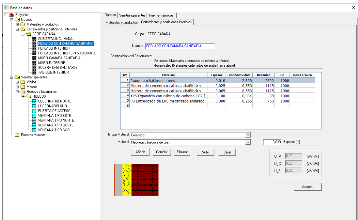
Imagen del levantamiento en HULC. Pantalla de base de datos constructiva.
