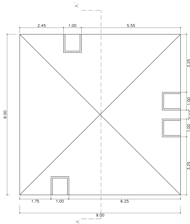
PLANTA CUBIERTA
