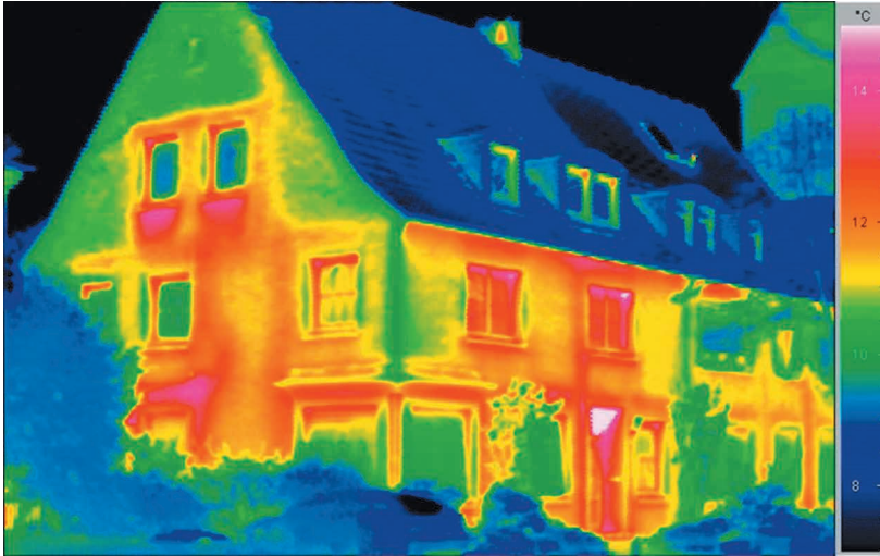
Figura 1. Pérdidas térmicas en un edificio residencial con un sistema deficiente de aislamiento. Fuente: Verband Privater Bauherren e.V./Bundesverband Deutscher Baustoff-Fachhandel e.V.
