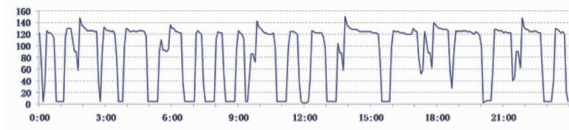
Figura 9. Perfil de consumo de una cámara de frío en la prueba de un simulador de temperatura de producto. Fuente: Enefyg-Ecoinversol.
