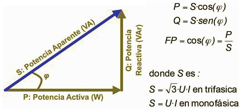
Figura 1. Triángulo de potencias. Fuente: RTR Energía.
