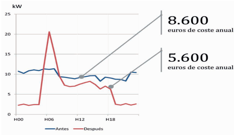
Figura 8. Diferencia de perfiles de consumo tras la adopción de una actuación en la climatización de un edificio. Fuente: Enefyg.
