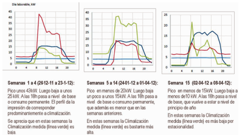
Figura 7. Evolución de los consumos semanales en una oficina. A partir de su estudio se van deduciendo oportunidades de ahorro. Fuente: Ecoinversol – Enefyg.
