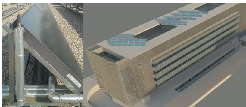
Figura 1. Imágenes de los módulos solares térmicos y de su disposición sobre la cubierta del edificio principal. Fuente: Elaboración propia.
