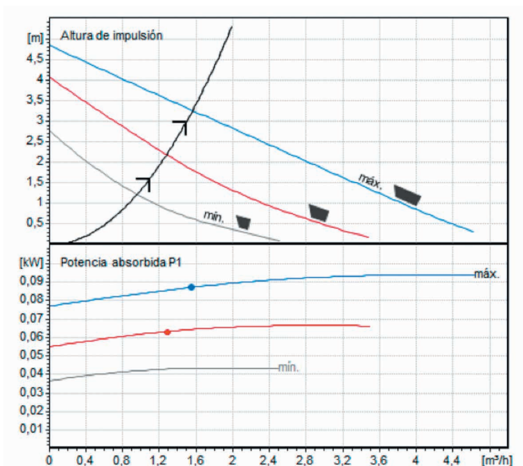
Figura 4. Circulador para ACS de 3 velocidades con motor asíncrono, seleccionado para un caudal de 1,5 m 3 /h a 3 m.c.a. y finalmente instalada para un caudal de 1,1 m 3 /h. Fuente: Elaboración propia.
