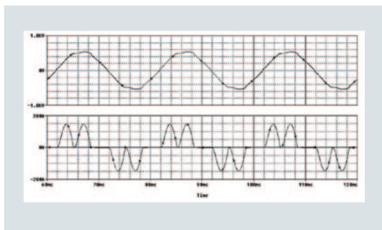
▫ Sin reactancia: THD=45%
