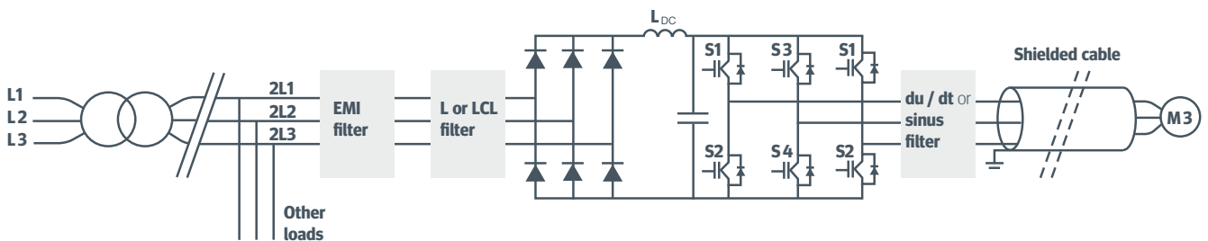
▫ Esquema de tipo de filtrado para convertidores trifásicos de potencia
