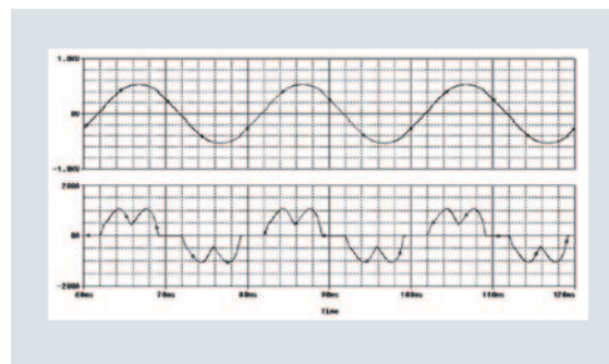
▫ Con reactancia: THD=20%
